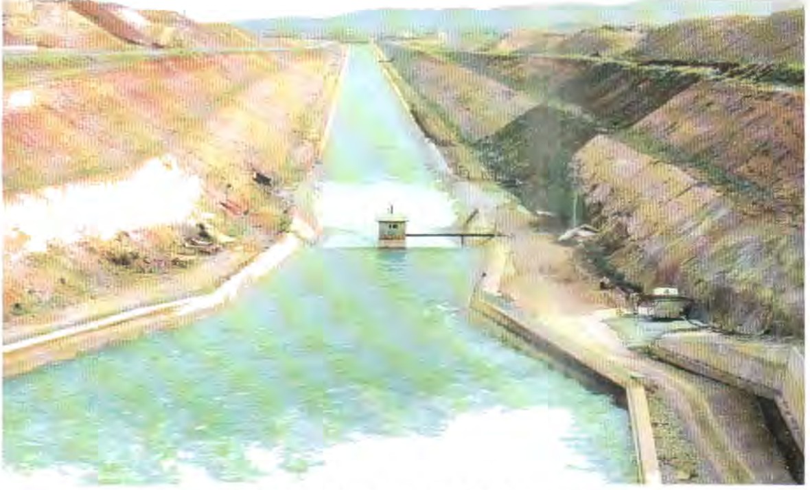
3) Fırat'ın sularını Harran'a kavuşturan Ana Sulama Sistemi
